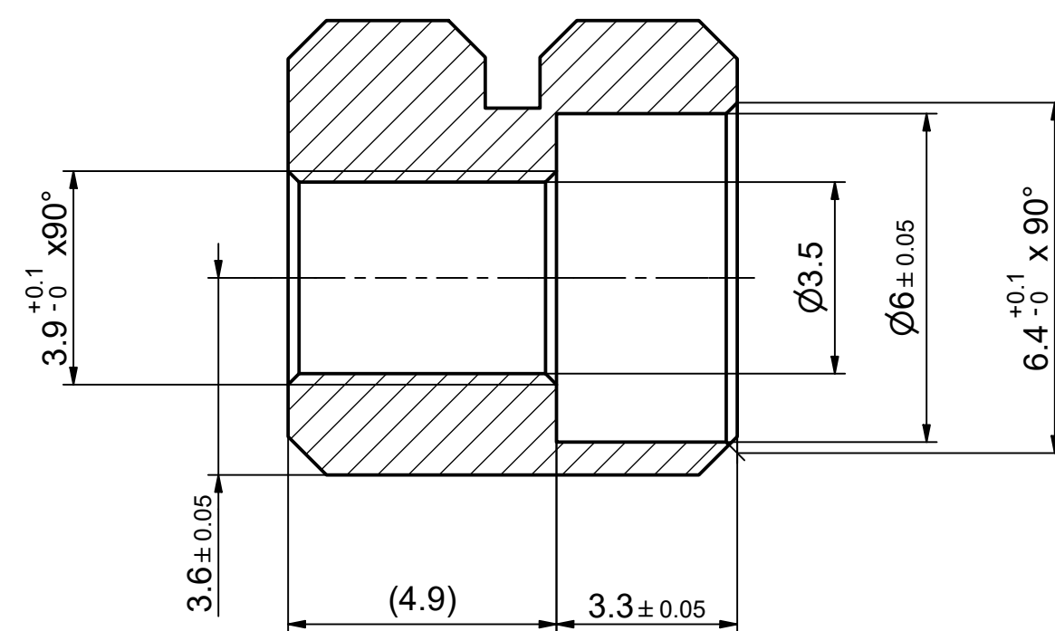
A-A (8 : 1)
