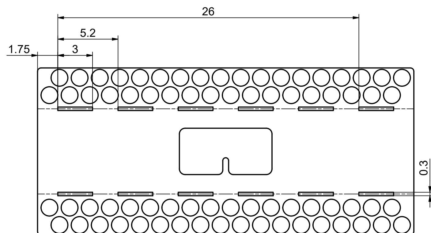
Abwicklung ( 5 : 1 )
