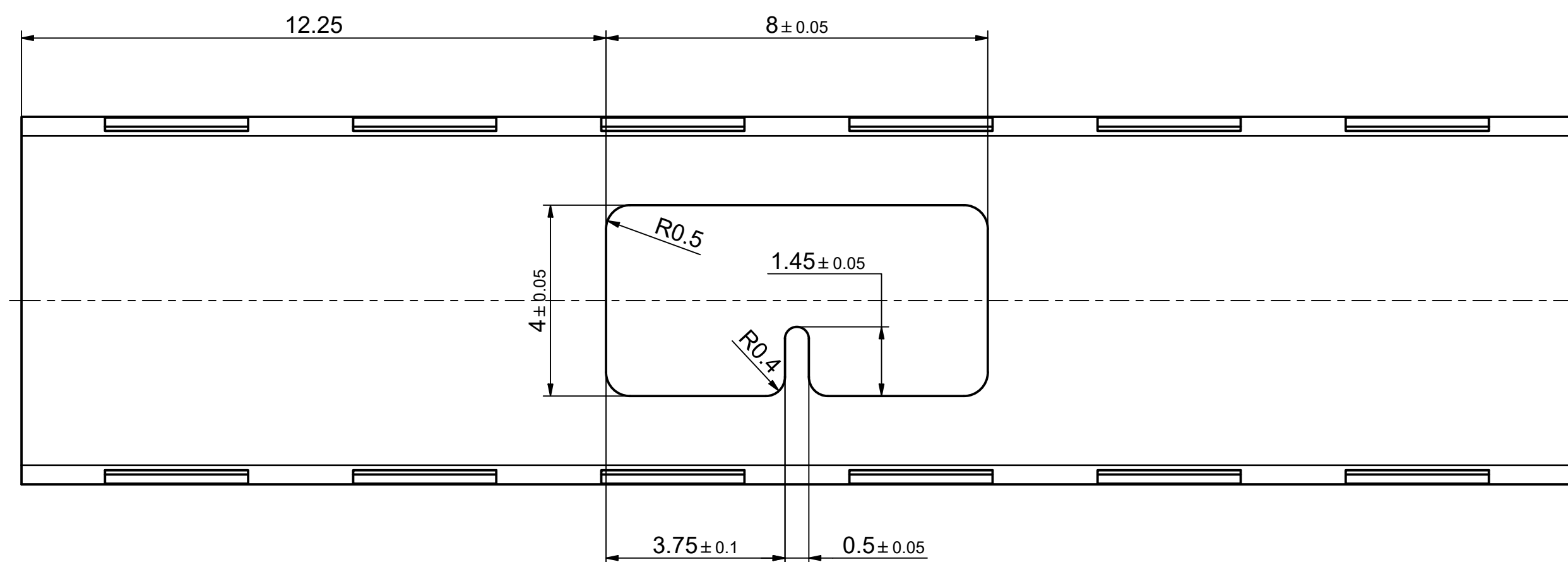
Abwicklung ( 5 : 1 )
