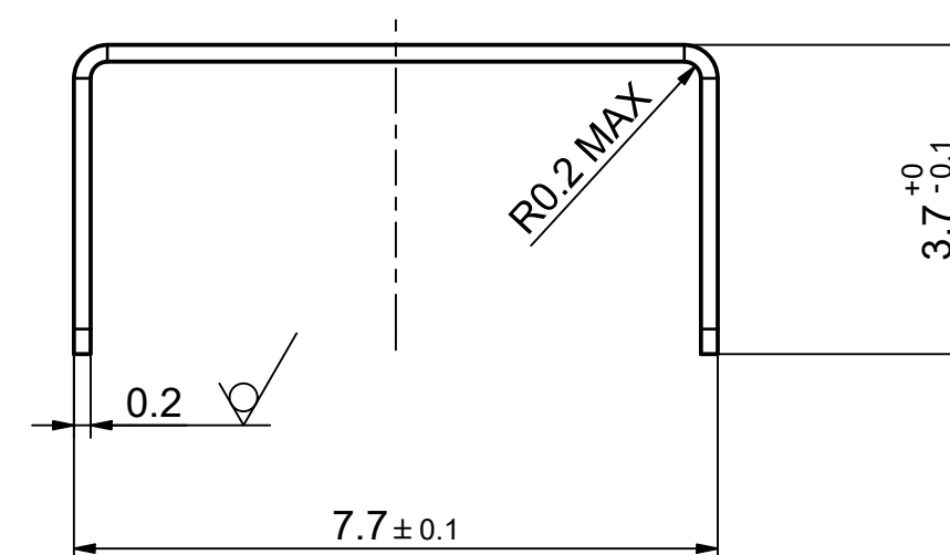
X ( 20 : 1 )
